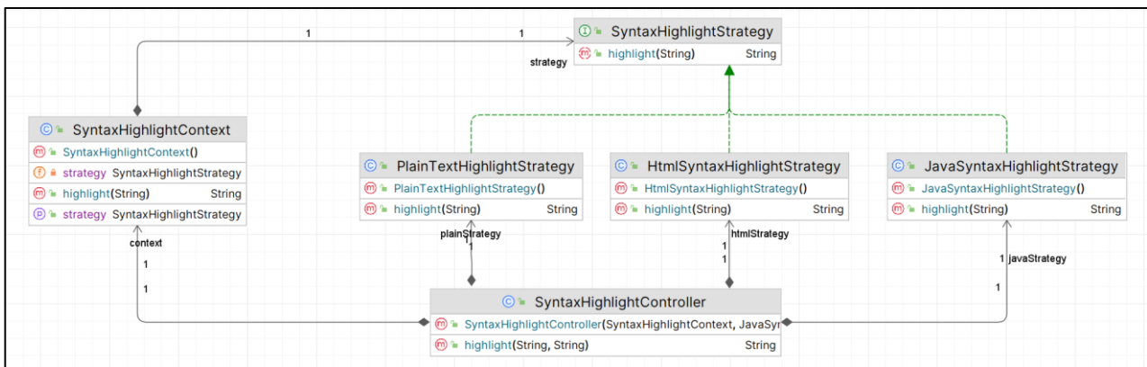
Рисунок 8. Діаграма класів для патерну «Strategy».
